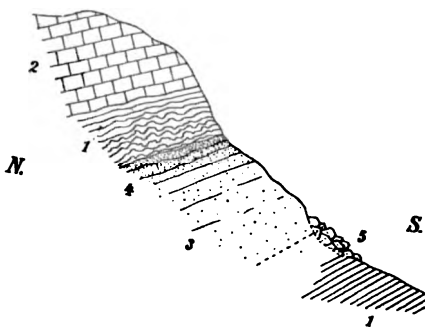
Fig. 1. Profil durch den Quarzporphyr- und Phyllitkontakt im Stojičevac dol auf der Südseite des Vratnica-Gebirges. 1 Karbonischer Phyllit. 2 Permo-karbonischer Kalkstein. 3 Quarzporphyr. 4 Derselbe in felsitischer Ausbildung. 5 Quarzporphyrschutt.
